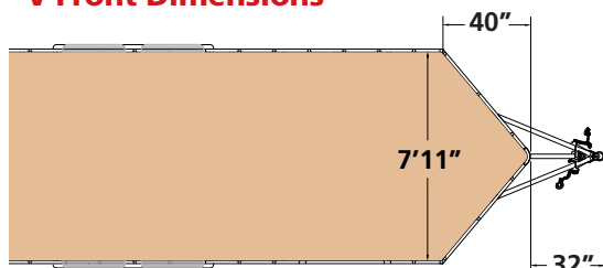
V-Front Dimensions
